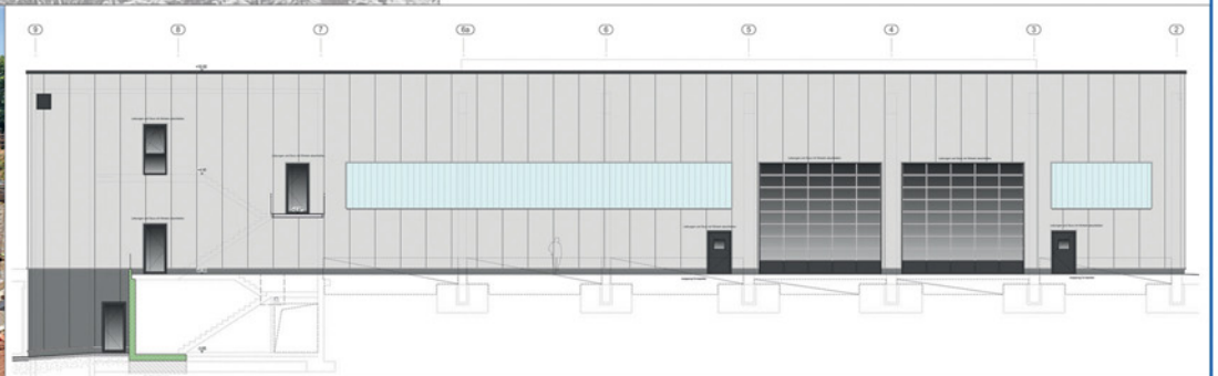
Ansicht Werkhalle von Norden
