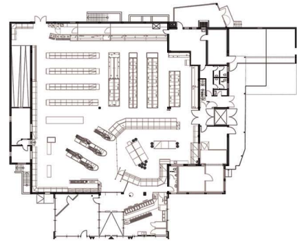
Grundriss Erdgeschoss
