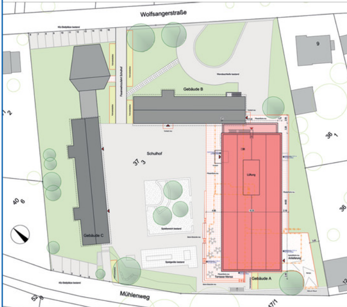
Freiflächenplan
