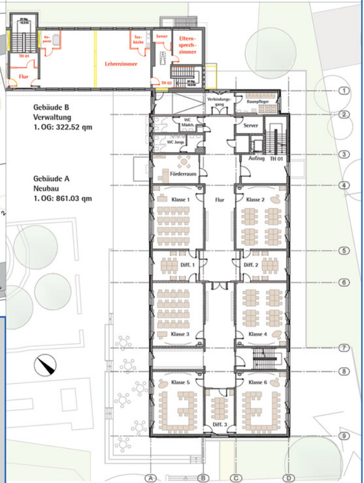
Grundriss 1. OG - Neubau mit Anschluss an Gebäude B
