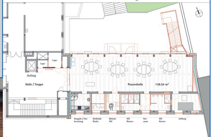
Grundriss Erdgeschoss - Pausenhalle
