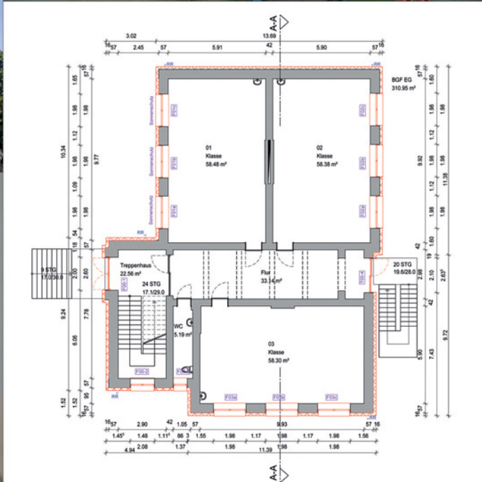
Grundriss Erdgeschoss
