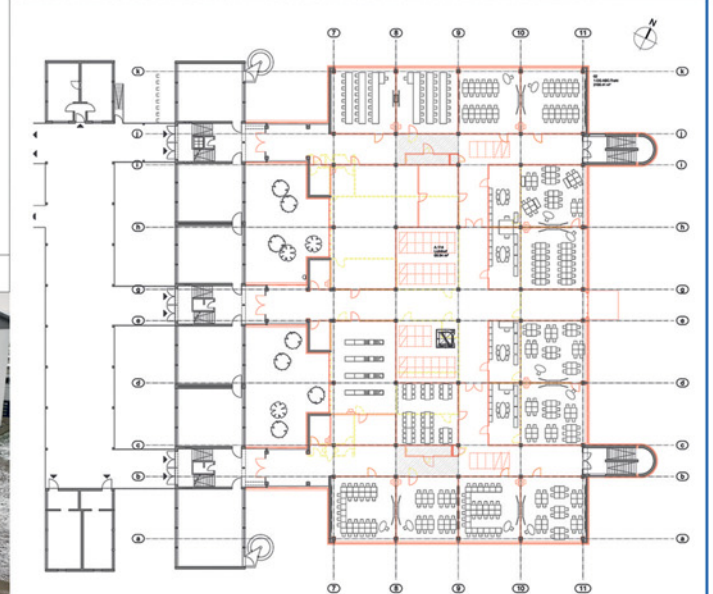
Grundriss 1. Obergeschoss - Werkplanung
