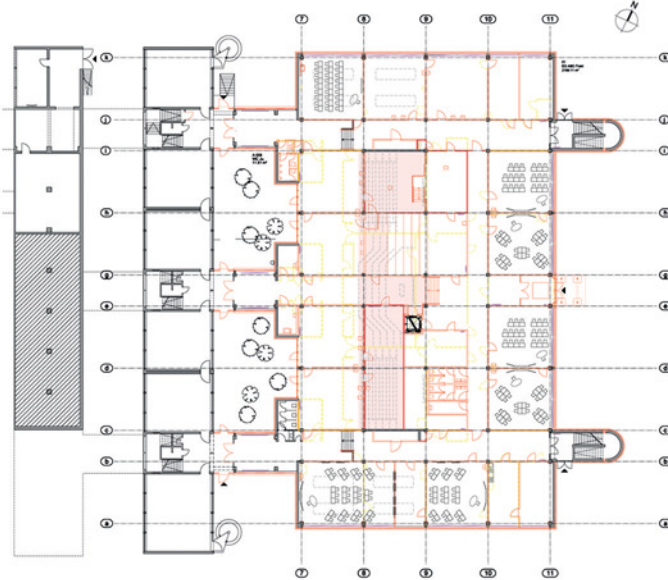
Grundriss Erdgeschoss - Werkplanung
