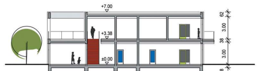
Schnitt A-A
